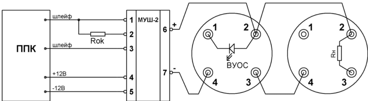
Схема подключения извещателей СПД-3 к ППК посредством МУШ-2
