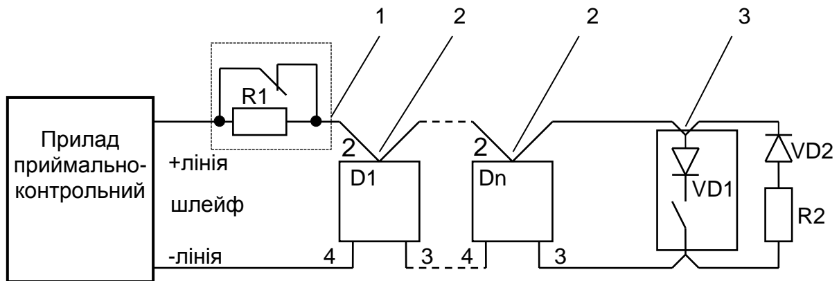
Рисунок 4. Схема підключення сповіщувачів у шлейф блока.
